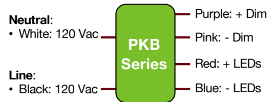
Wiring Diagrams
